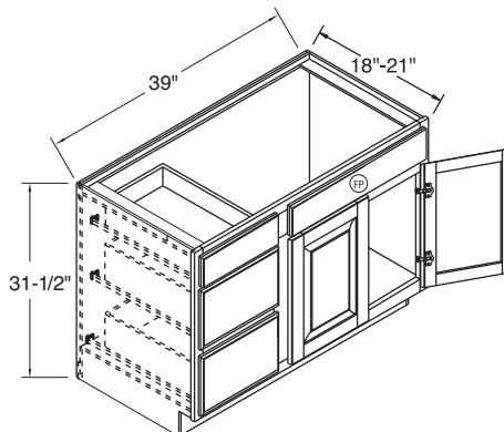
VBB3918D-VBB39D L or R
