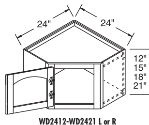
WD2412-WD2421 L or R
