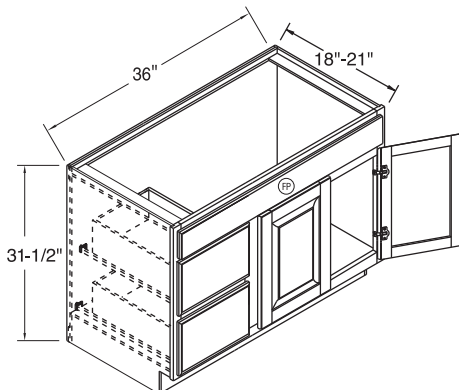
VBB3618D-VBB36D L or R
