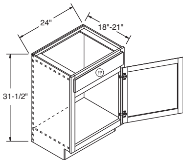
VSB2418-VSB24 L or R
