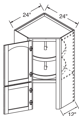
WDD2448S-WDD2454S L or R
